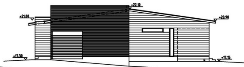
JULKISIVU LÄNTEEN
